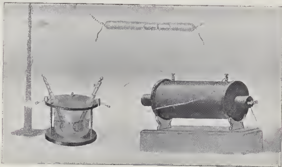
Apparato trasmettente e coherer.
